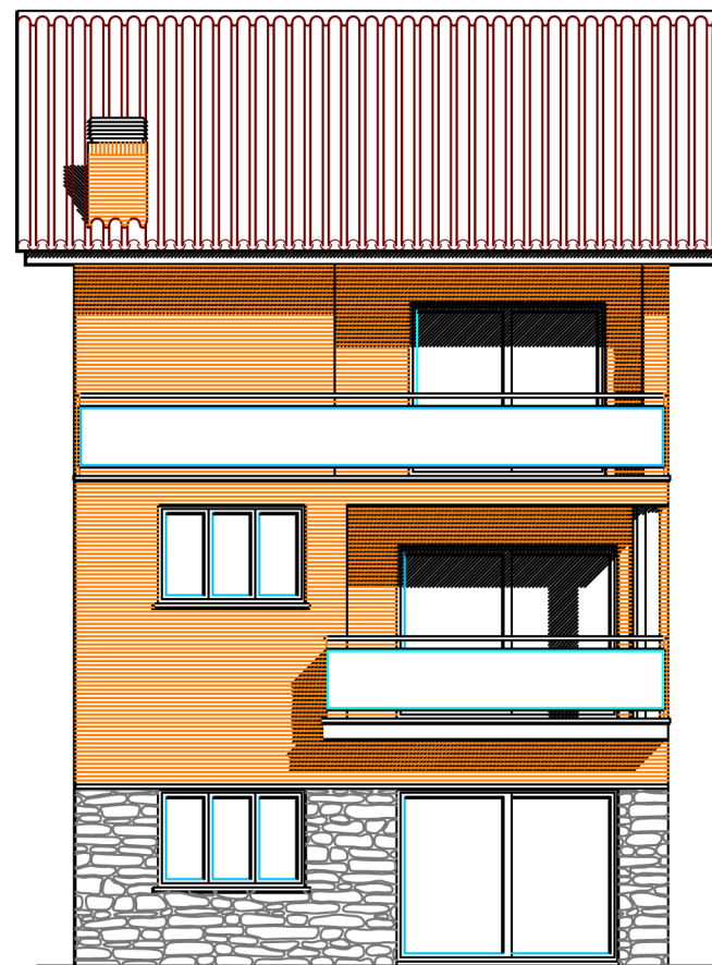
FAÇANA A-B
